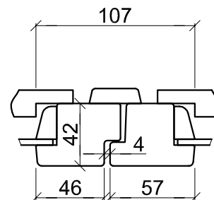
Pool-poollega raamid
