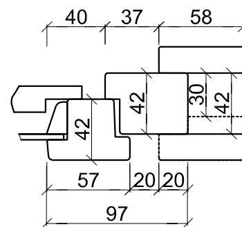
Avatav aken
