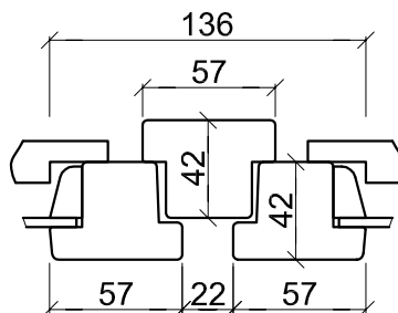
Impostiga
